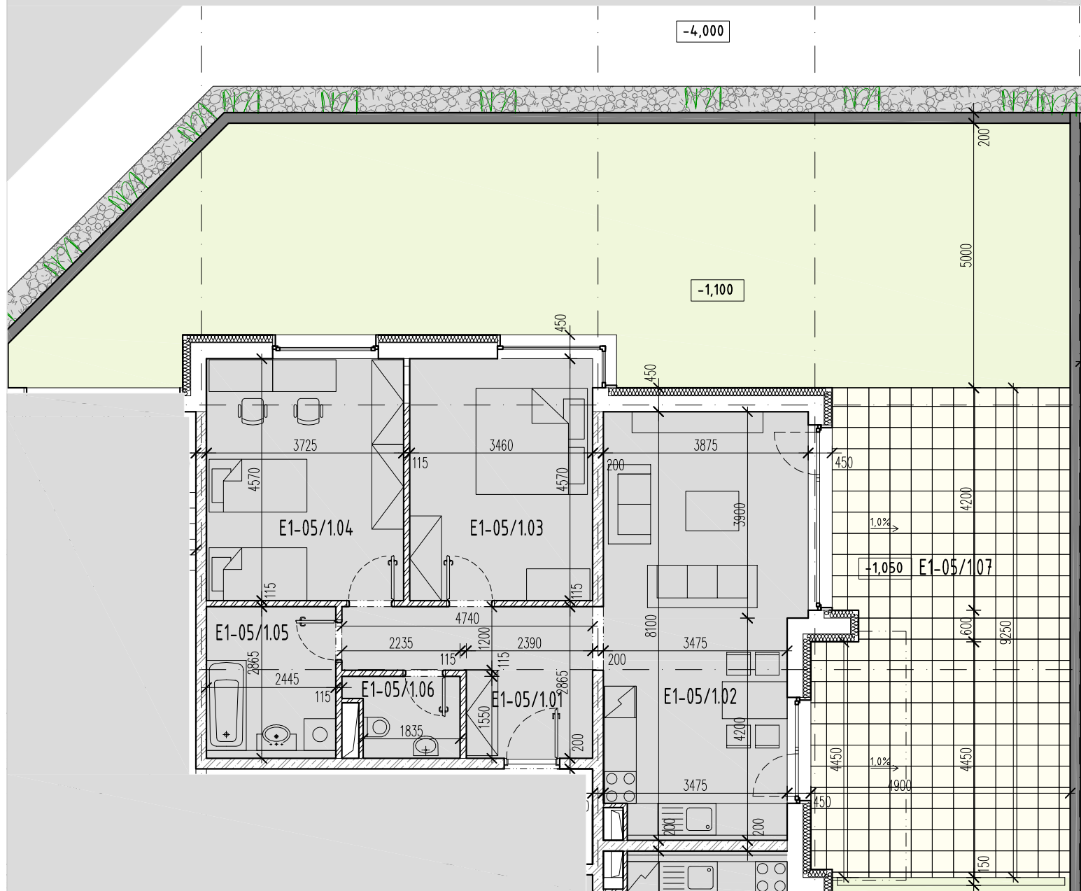
PÔDORYS BYTU GROUNDPLAN
